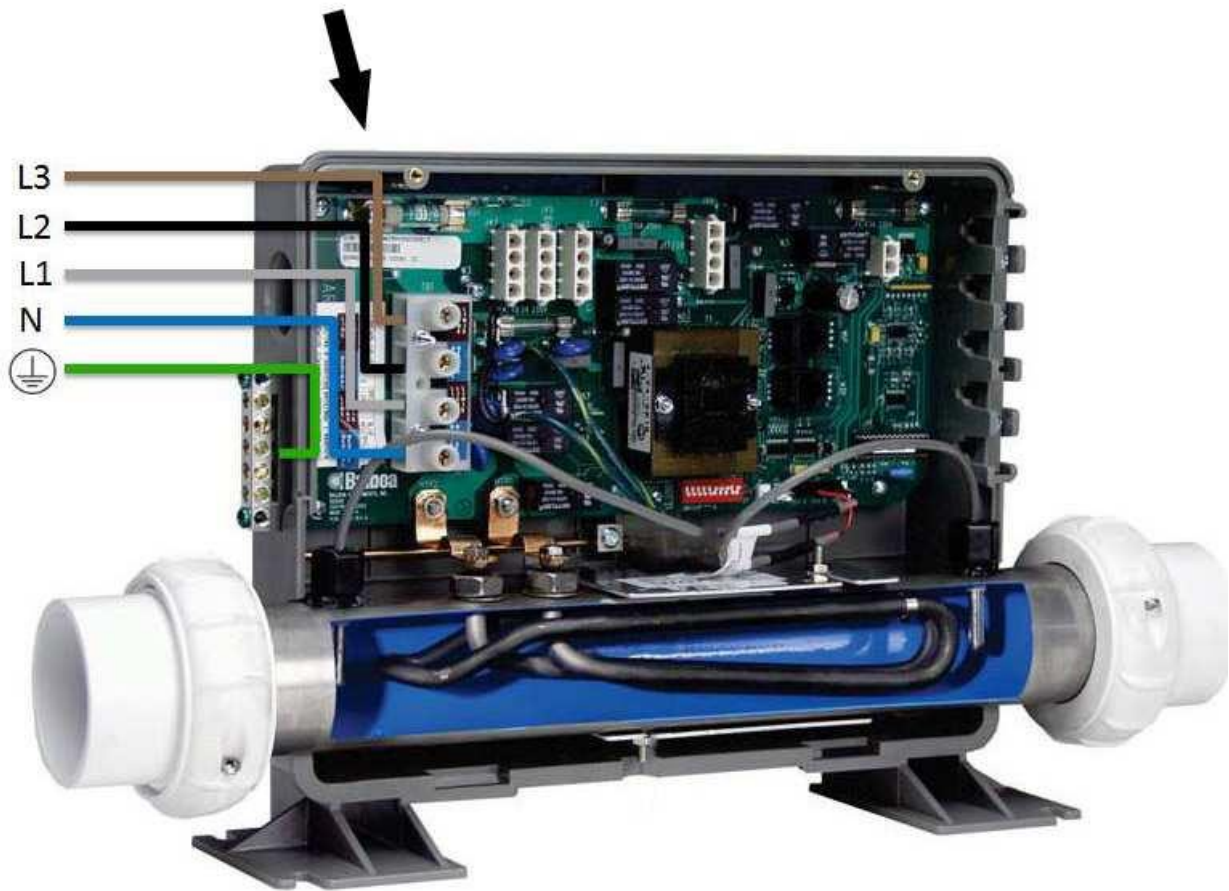
Bild 2: Märkningens plats på styrenheten.
